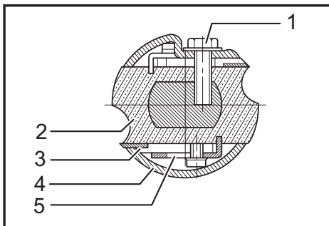
► 1. Pernos 2. Tambor 3. Cuchilla del cepillo 4. Cubierta del tambor 5. Placa de ajuste
