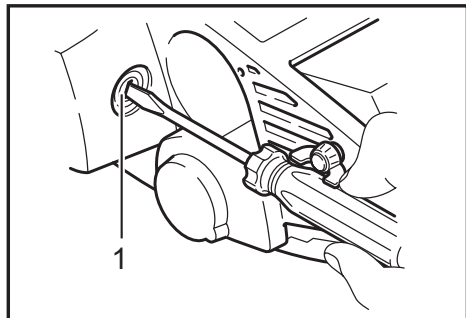
► 1. Tapa del carbón
