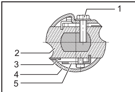
► 1. Boulons 2. Bloc de coupe 3. Fer de rabot 4. Contre-fer 5. Plaques de réglage
