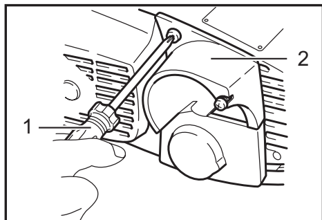
► 1. Tournevis 2. Couvercle à copeaux
